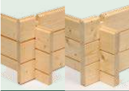
Eckversatz 28/40 mm Bohlen
