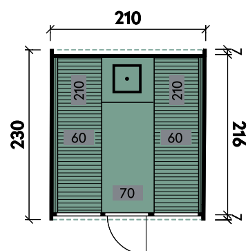
Carol 2123 Gerade Liege
