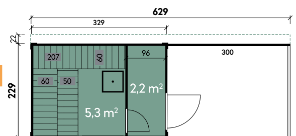
Sidonia 6323 2-Raum | Seitendach 3 m
